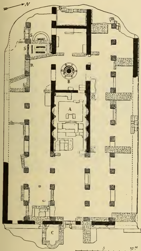
10505. — Plan de la basilique chrétienne de Cumès. D'après Atti del III congresso internazionale di arch. crist. , 1932, Rome, 1934, p. 227, fig. 3.
